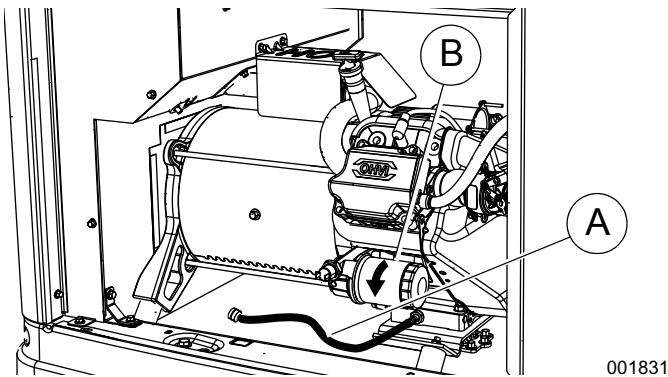
Figure 4-2. Emplacement du filtre à huile et du tuyau de vidange (9 kW)
