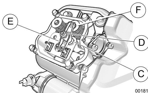
Figure 4-7. Réglage du jeu des soupapes (9 kW)
