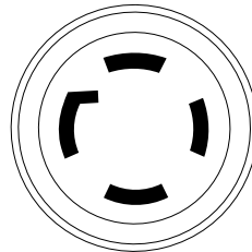
Figura 2-5. Toma de corriente de 120/240 VCA, 30 A NEMA L14-30
