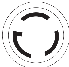
Figure2-6. Prise 120 V CA, 30 A NEMA L5-30
