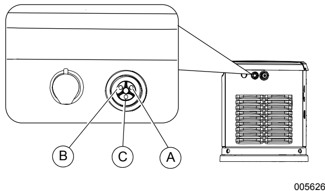
Рис. 3-3. Светодиодные индикаторы
