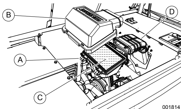
Рис. 4-4. Обслуживание воздухоочистителя
