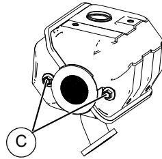
Figura 4-11. Sujetadores del parachispas
