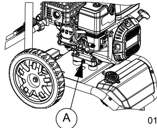
Figure 4-7. Bouchon de vidange d'huile
