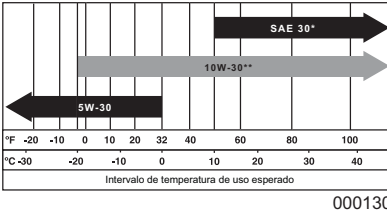
Figura 4-4. Viscosidad del aceite
