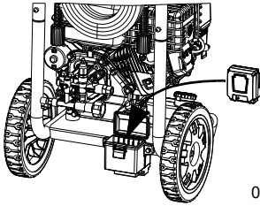
Figura 2-7. Instale la batería
