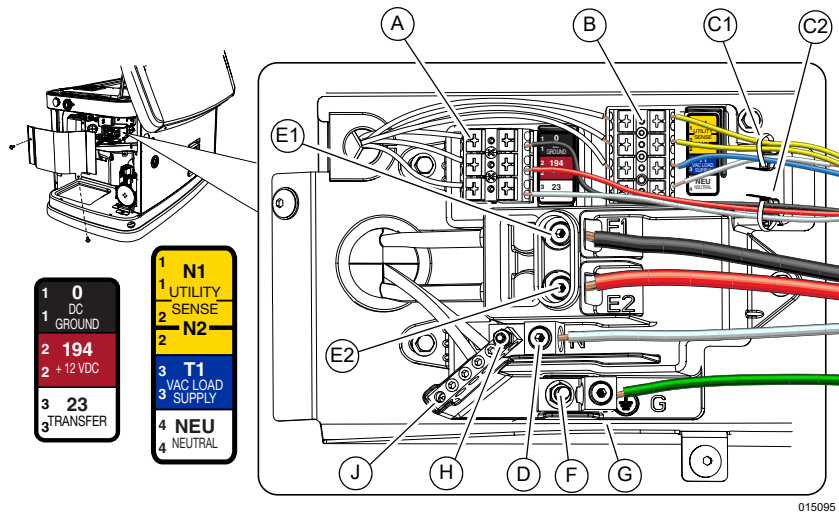
Figura 6-1. Conexiones del cableado eléctrico
