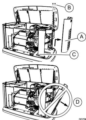
Figura 2-6. Retiro del panel lateral de entrada
