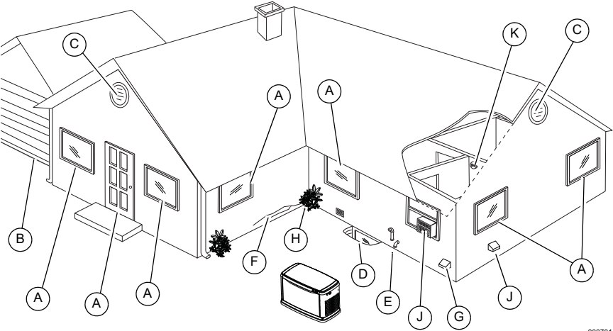
Figura 3-1. Monóxido de carbono—Posibles puntos de entrada
