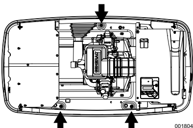
Figura 4-2. Ubicaciones de los orificios de montaje
