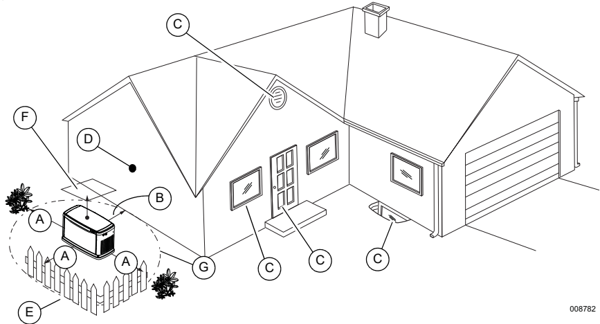
Figura 3-2. Requisitos de distancia del generador
