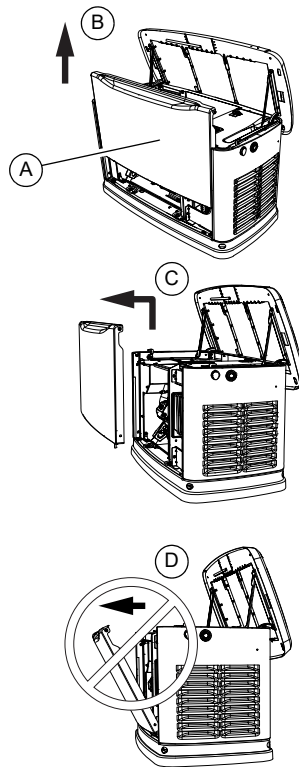
Figura 2-5. Retiro del panel de acceso delantero
