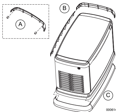
Figura 4-3. Instalación de la carcasa
