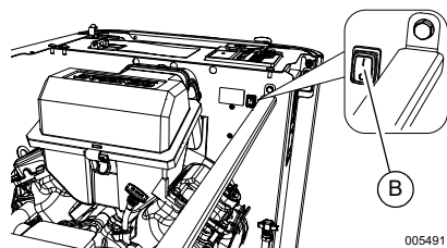
Figura 2-12. Interruptor de desconexión de emergencia (14 a 26 kW)
