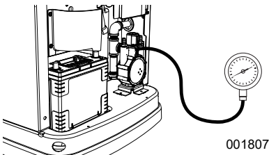
Figura 5-4. Revisión de la presión con manómetro
