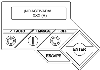
Figura 7-2. Pantalla No activada
