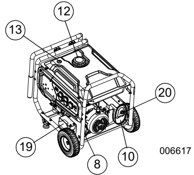
Figura 2-1. Controles y funciones
