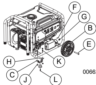
Figure 2-10. Montage des roues et du châssis
