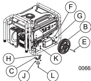
Figura 2-10. Conjunto de ruedas y patas
