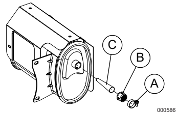
Figure 4-6. Filtre du pare-étincelles
