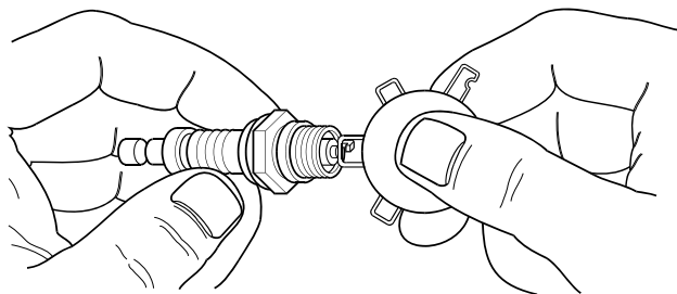
Figura 16 - Espaciamento de la bujía
