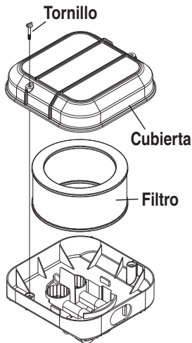
Figura 4.5 — 14, 17 y 20kW Limpiador de aire del motor
