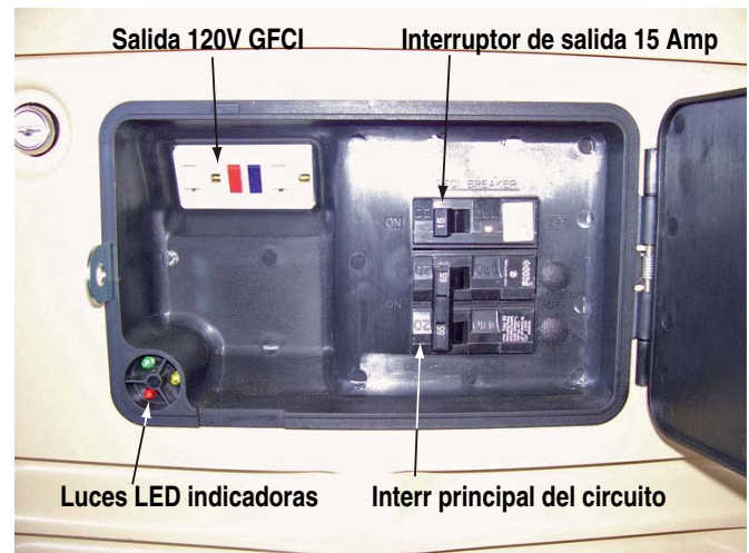
Figura 3.4 – Compartimiento lateral abierto
