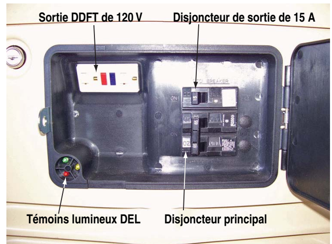
Schéma 3.4 – Compartiment latéral ouvert
