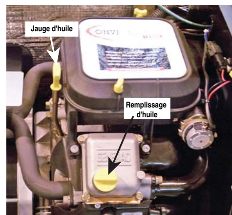
Schéma 4.3 — Jauge et remplissage d'huile, 14, 17 et 20 kW
