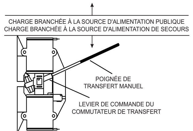
Schéma 3.2 – Fonctionnement manuel du commutateur de transfert
