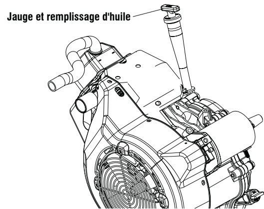
Schéma 4.2 — Jauge d'huile, 10 kW
