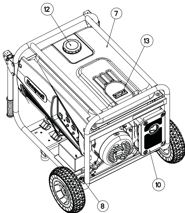
Figura 4 - Controles del generador
