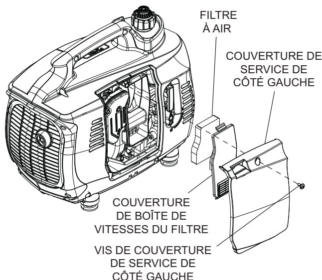
Figure 10 - Filtre à air
