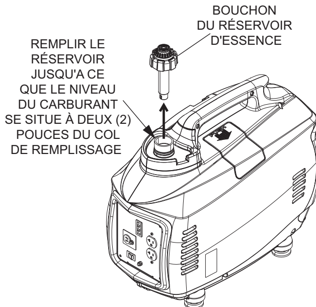
Schéma 8 - Bouchon du réservoir d'essence
