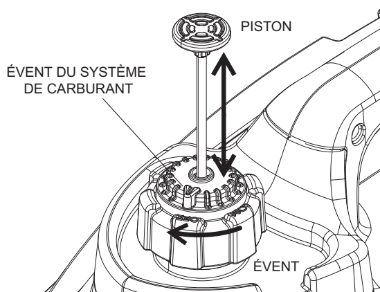
Schéma 5 - Amorçage du système de carburant
