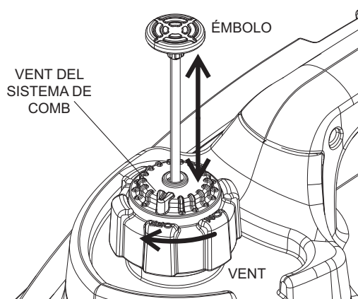
Figura 5 - Purgar sistema de combustible
