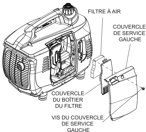
Schéma 10 - Filtre à air
