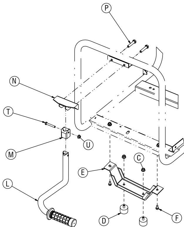
Рисунок 1С. Сборка ножки (GP5000/GP6000)
