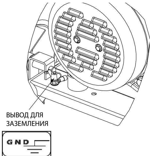
Рисунок 8. Заземление генератора
