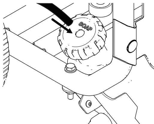
Figure 23 — Installer le tube de siphonnement
