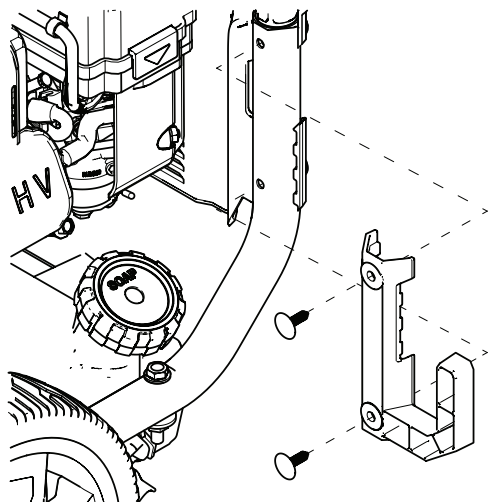
Figure 3 — Fixer le crochet de la lance à l'appareil
