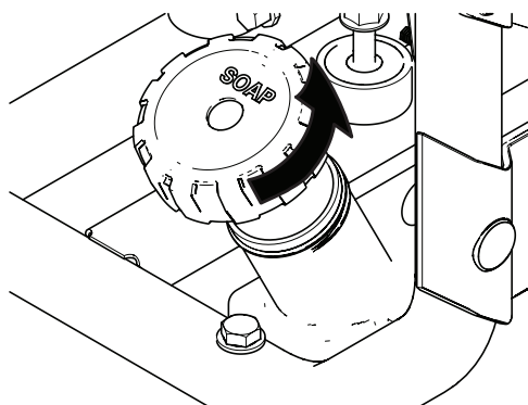
Figure 34 — Bouchon/tuyau de siphonnement de produit chimique
