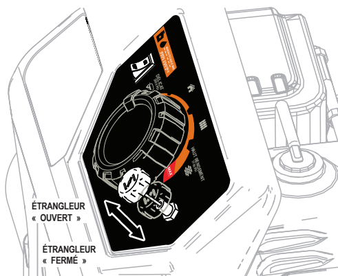
Figure 30 – Bouton de l'étrangleur
