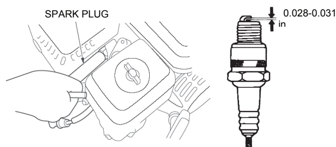
Figure 42 — Changer la bougie d'allumage
