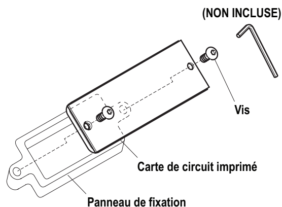
Figure 32 — Carte de circuit imprimé
