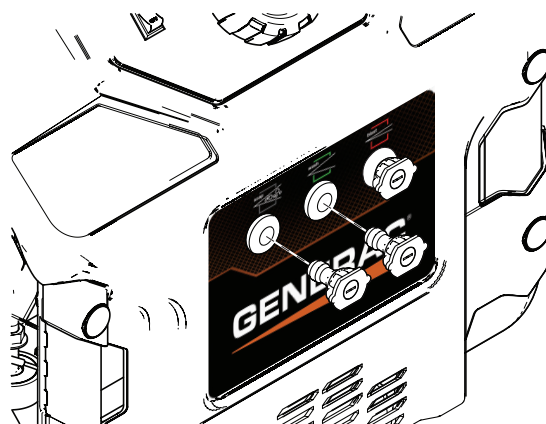
Figura 6 - Inserción de las boquillas
