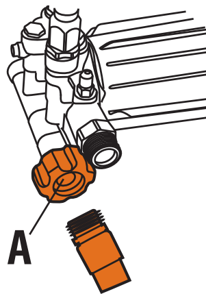
Figure 11 — Inspecter le tamis de l'entrée d'eau
