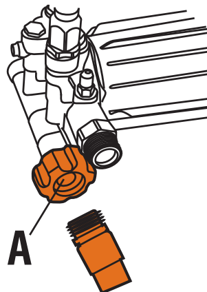
Figura 11 - Inspección del colador de entrada
