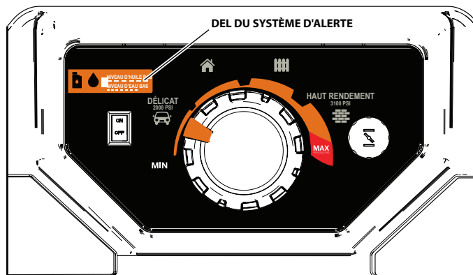
Figure 25 – DEL du système d'alerte
