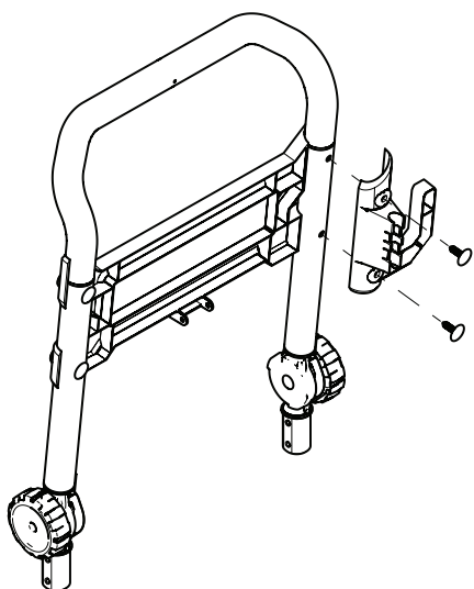
Figure 2 — Fixer le crochet du pistolet à l'ensemble de la poignée
