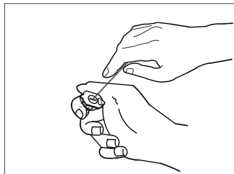
Figure 36 — Retirer un corps étranger
