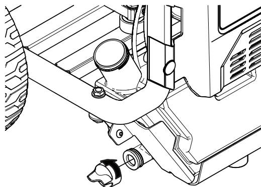
Figure 35 — Bouchon du drain du réservoir de produits chimiques
