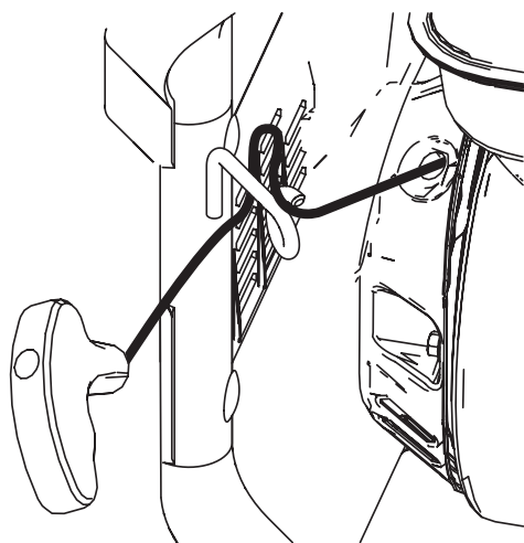
Figure 8 — Crochet de la corde du lanceur à rappel
