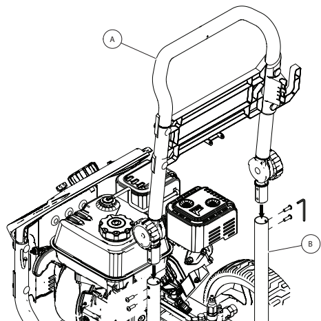
Figure 4 — Fixer la poignée à l'appareil
