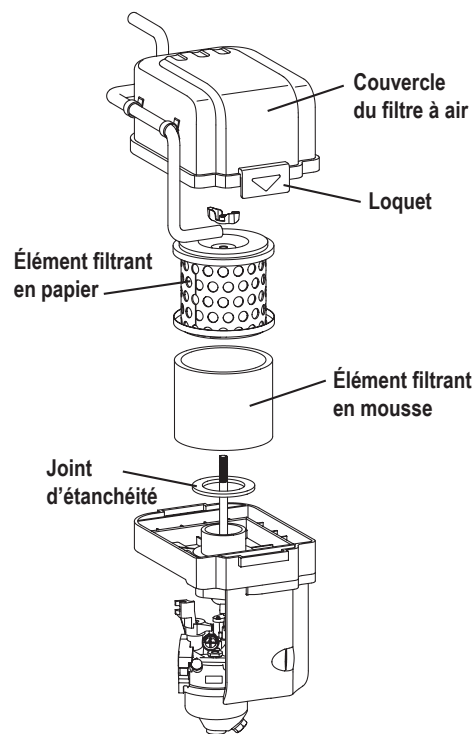
Figure 41 — Nettoyer le filtre à air
