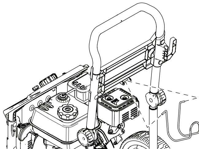
Figure 5 — Installer le crochet du tuyau
