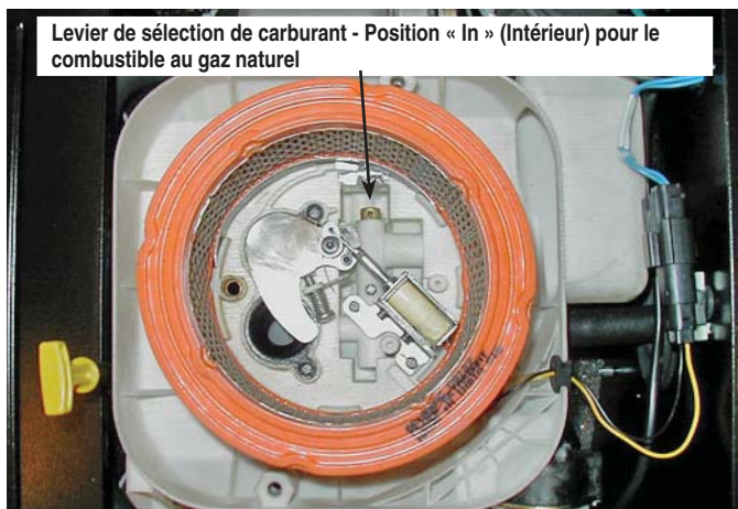
Figure 1.8 - GT-990/GT-999, 13, 14, 16, 17 et 20 kW (couvercle de boîte à vent retiré)
