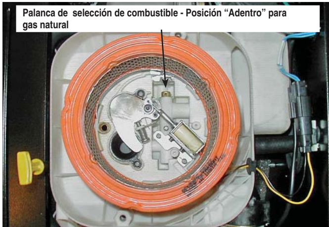
Figura 1.8 - 13, 14 y 16 kW, GT-990/GT-999 (cubierta de caja de aire retirada)
