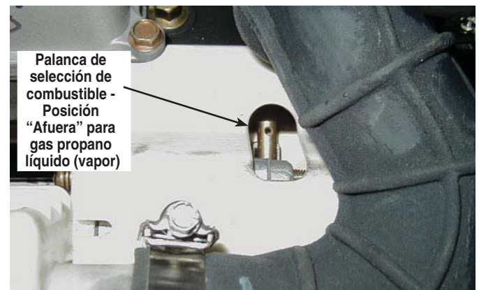
Figura 1.6 - 10 kW, GT-530 (manguera de entrada deslizada atrás)
