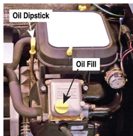
Figura 4.3 — Varilla de aceite y llenado, 13, 14, 16, 17 y 20 kW
