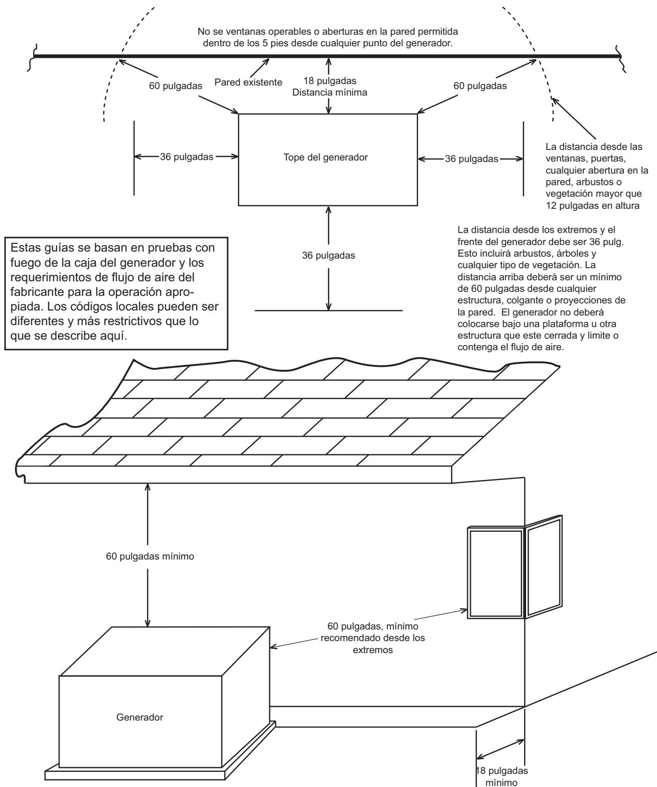
Figure 1.10 – Lineamientos de instalación
