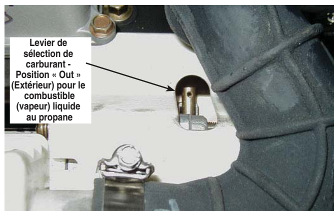
Figure 1.6 - GT-530, 10 kW (remise du tuyau d'admission)
