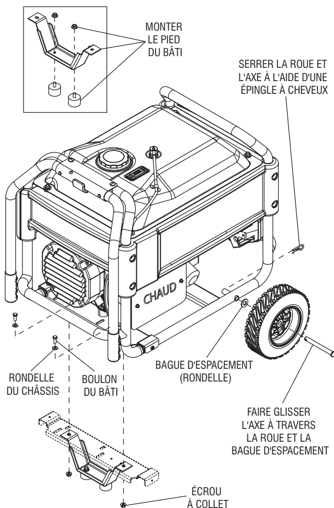
Schéma 2 – Montage des roues et du pied
