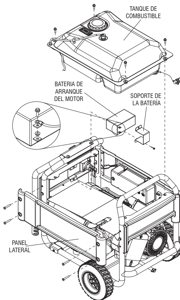
Figura 16 – Extracción de la batería
