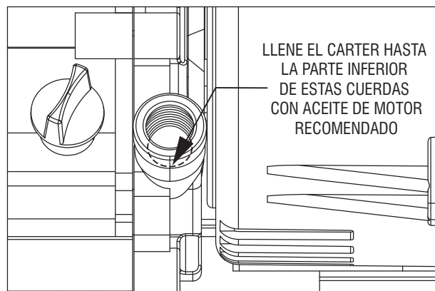
Figura 8 – Nivel de aceite
