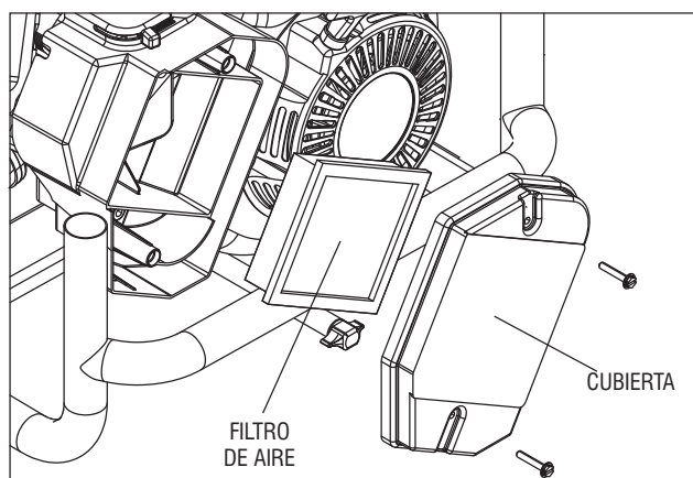
Figura 13 - Filtro de aire
