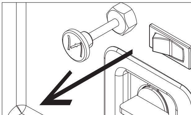
Figura 11 – Operación del choke
