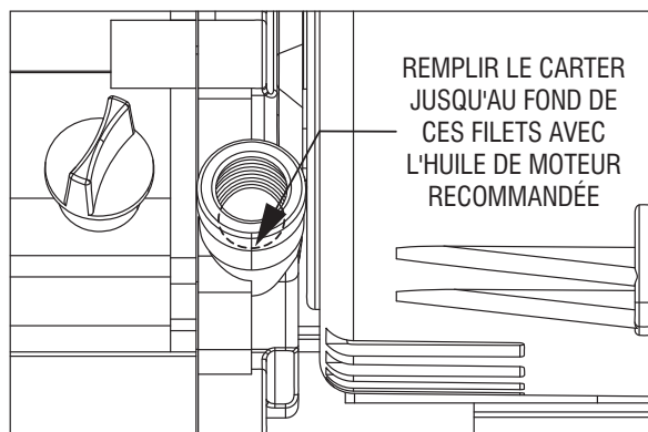
Schéma 8 – Niveau d'huile
