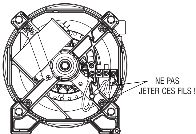
MISE À LA TERRE DU CONDUCTEUR NEUTRE AU CHÂSSIS
