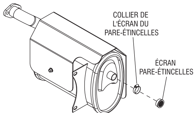
Schéma 14 – Écran pare-étincelles
