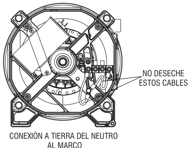
Figura 7 – Conexión a tierra de neutro a marco
