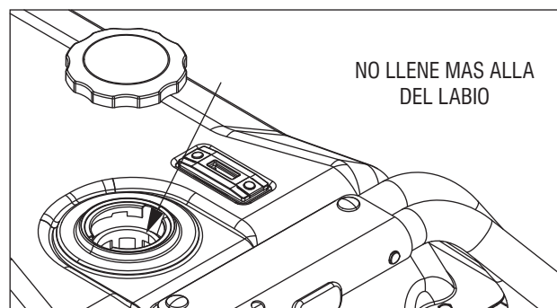
Figura 9 – Nivel de llenado de combustible
