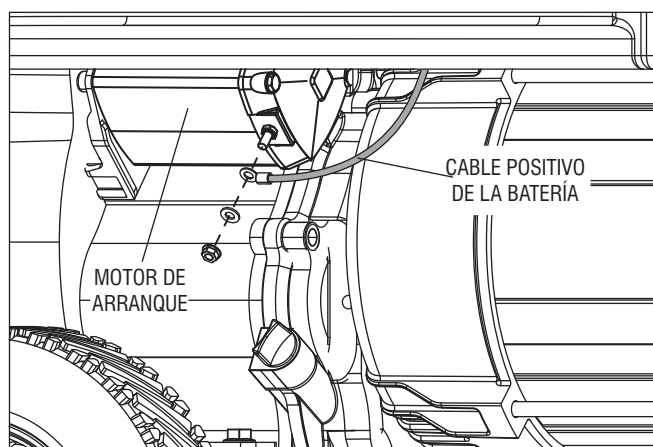
Figura 4 – Conexión de la batería
