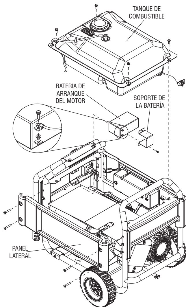
Figura 16 – Extracción de la batería
