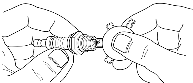
Schéma 12 – Écartement de la bougie d'allumage
