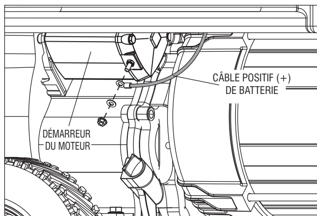
Schéma 4 – Branchement de la batterie
