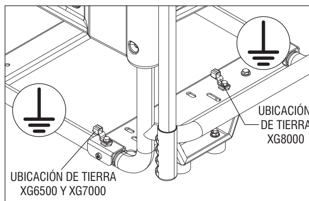
Figura 6 – Ubicaciones de la tierra del generador
