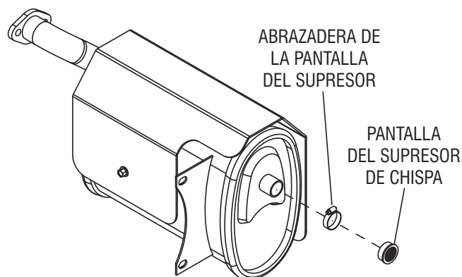
Figura 14 – Pantalla del supresor de chispas
