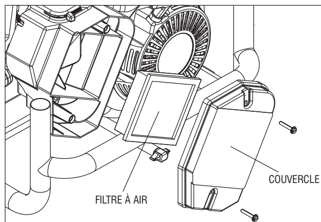
Schéma 13 – Filtre à air
