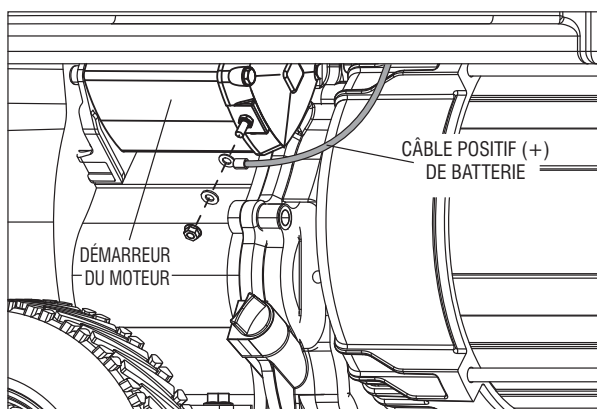
Schéma 4 – Branchement de la batterie
