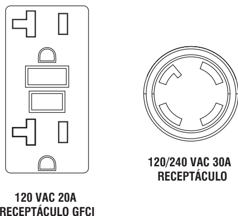
Figura 6 – Receptáculos del generador
