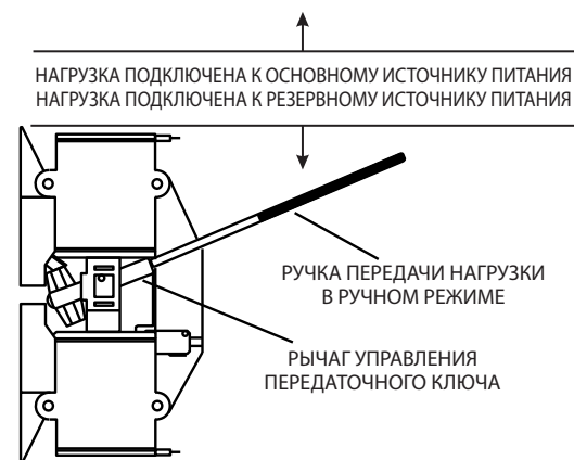
Рисунок 3.2 – Работа передаточного ключа в ручном режиме
