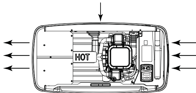
Figura 4.8 - Respiraderos de enfriamiento
