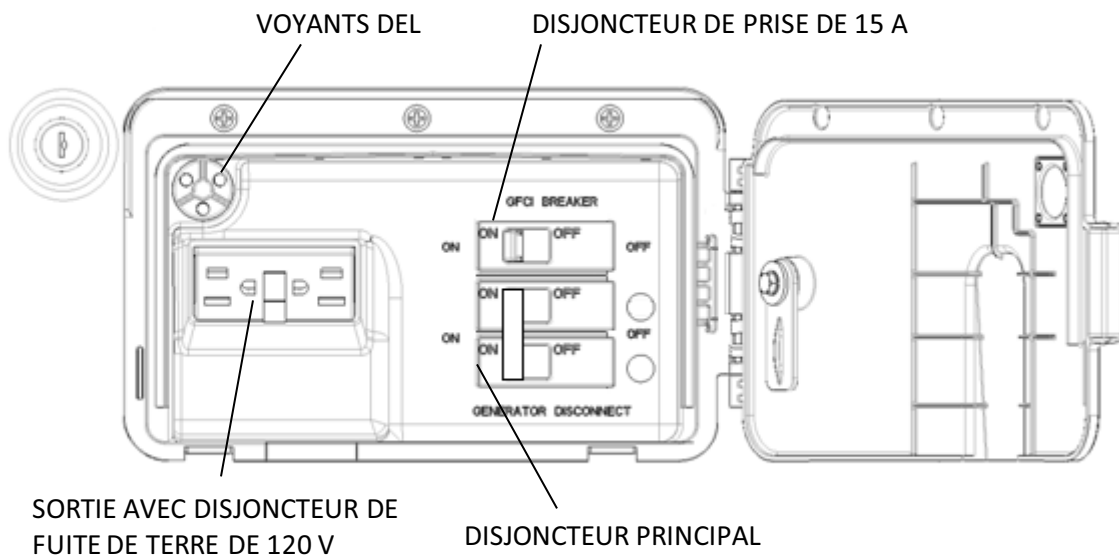
Figure 3-5 : Compartiment latéral ouvert
