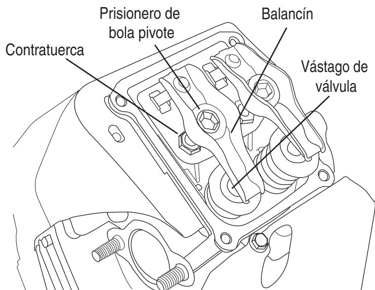
Figura 4-4: Ajuste de la luz de válvulas
