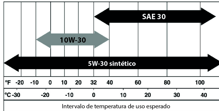
Figura 4-1: Aceite recomendado en base a la temperatura
