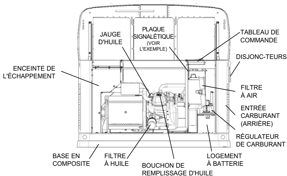
Figure 2-1 : Moteur GH-410, appareil de 8 kW
