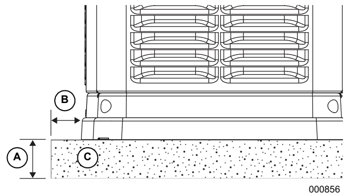
Figura 3-3. Base de gravilla compactada
