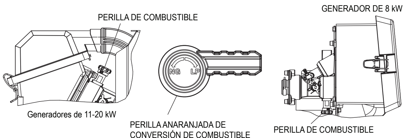
Figura 5.1 - Ubicación de la perilla de conversión de combustible para generadores de uno y dos cilindros
