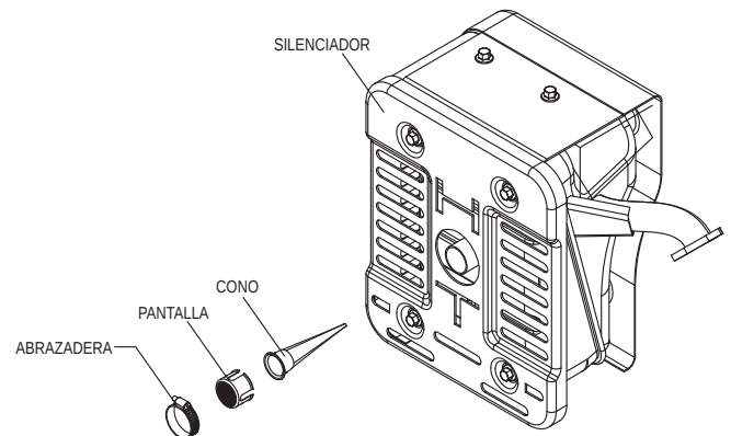
Figura 16 - Supresor de chispas
