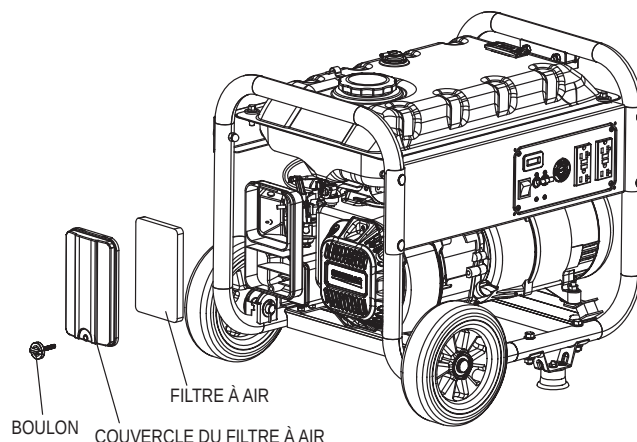
Figure 17 – Filtre à air
