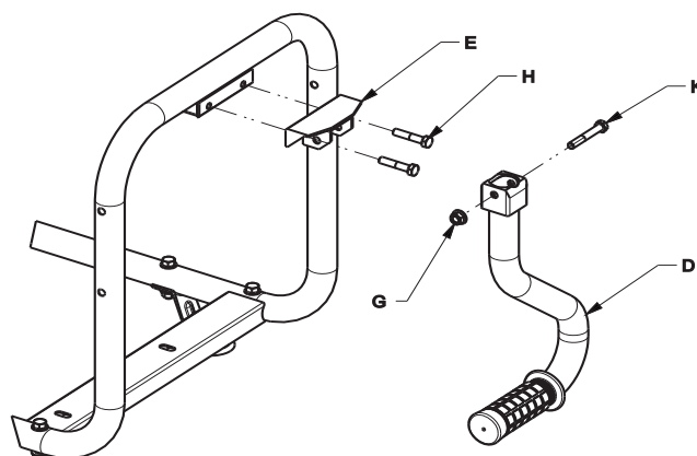
Figure 2 – Kit de la poignée
