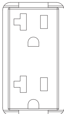
Figura 6 - Tomacorriente doble de 120 VCA, 20 A
