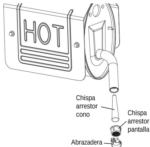
Figura 17 – Tamiz del supresor de chispas
