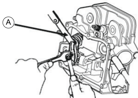
Figura 4-6. Ajuste de la holgura de la válvula
