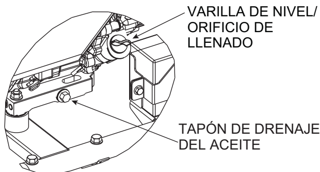
Figura 4-1. Tapón de drenaje trasero
