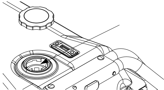
Figura 2-12. Nivel de llenado del combustible
