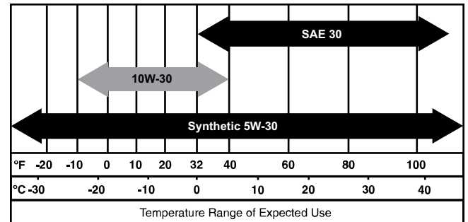
Figure 4-1. Huile recommandée en fonction de la température
