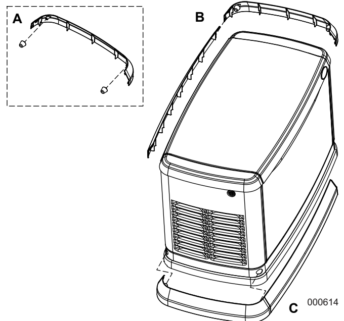
Figura 4-3. Instalación del frente
