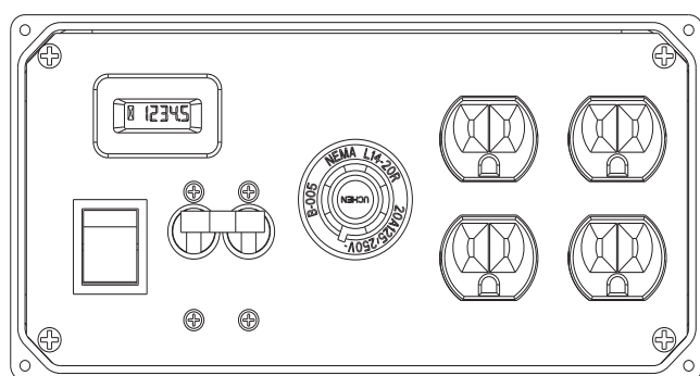
Figure 8 – Prise de courant double de 120 V c.a. et Prise à verrouillage de 120/240 V c.a.
