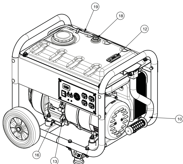
Figure 5 – Commandes du générateur
