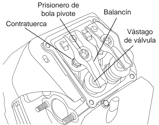
Figura 18 - Ajuste de la luz de válvulas
