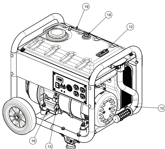
Figura 5 - Controles del generador
