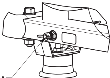
Figura 9 - Conexión a tierra del generador
