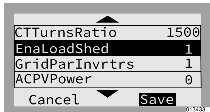
Figura 7-21. PV + Almacenamiento: Todo el hogar (3 de 3)
