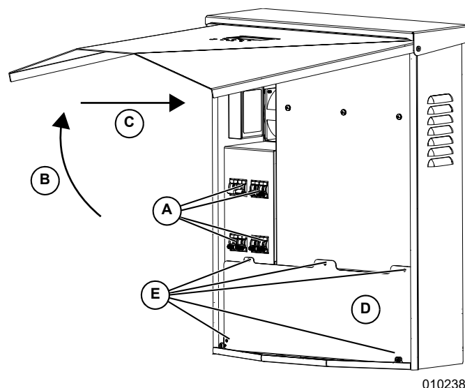
Figura 8-1. Compartimiento de cableado
