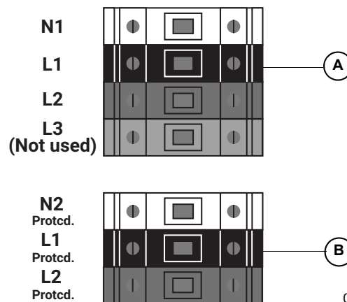
Figura 5-7. Terminales de cableado de CA
